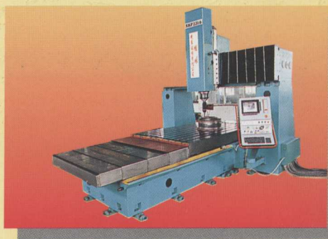
XKF2316 数控龙门仿形铣床
