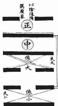
随卦係失图
