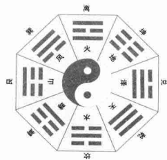
文王八卦图
