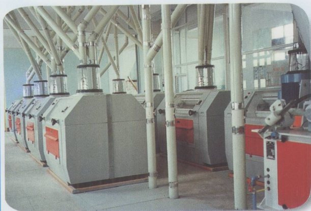
▲ 1987 年汕头市面粉厂引进的意大利面粉生产设备
