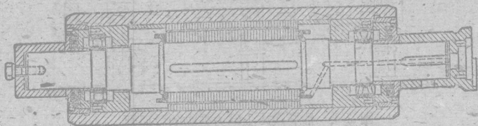
圖 1-12 轉子在外面的電動機滾子。
