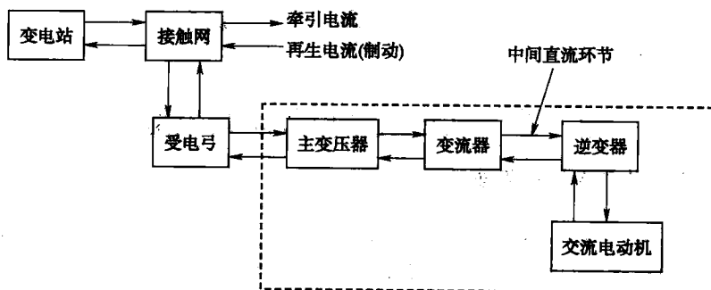
图 1-2 交—直—交牵引传动系统构成
