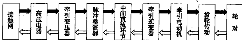
图 1-3 能量变换与传递途径示意图
