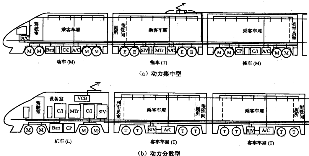
图 1-4 动力配置形式
