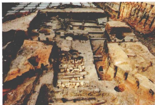
南越国木构水闸遗址。
