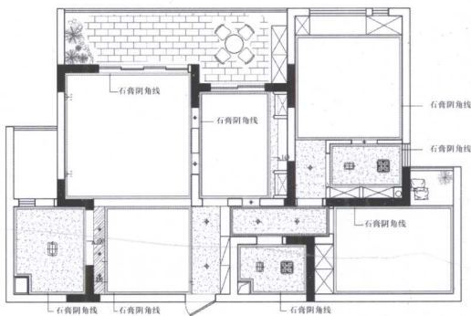
平面布置图
