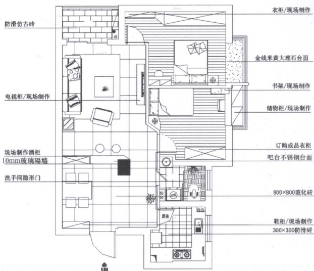
平面布置图
