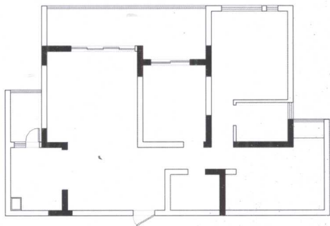
原始平面图
