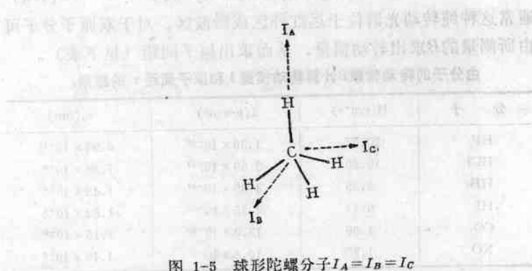
图 1-5 球形陀螺分子 I_A = I_B = I_C
