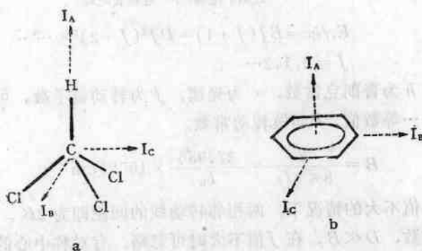
图 1-4 对称陀螺分子
