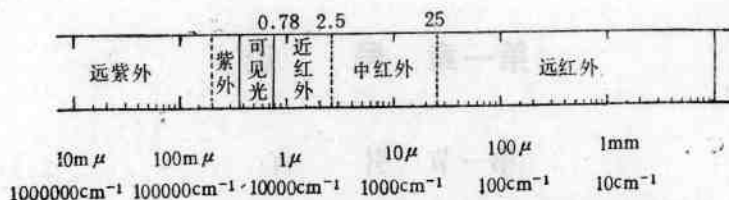
图 1-1 红外区的划分
