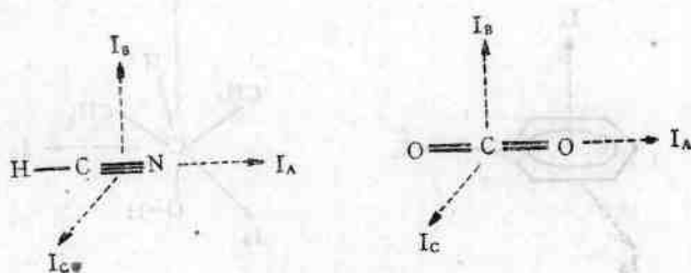
图 1-3 线性分子 I_A=0 I_B=I_C
