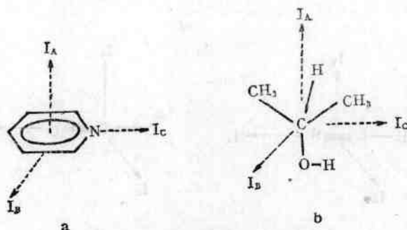
图 1-6 不对称陀螺分子 I_A < I_B < I_C a—近扁平陀螺; b—近狭长陀螺
