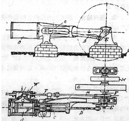
第81圖 單缸蒸汽機及其滑閥控制
