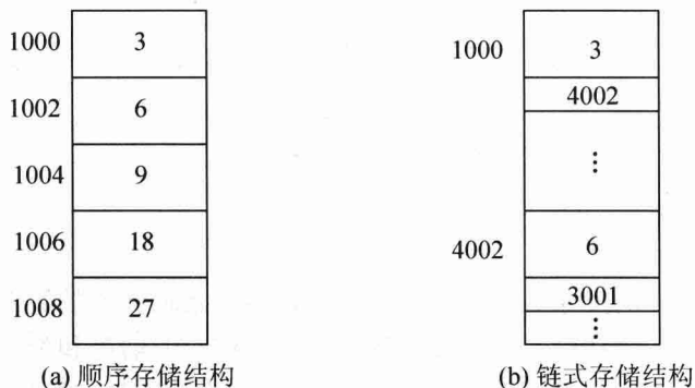
图 1.4 数据结构 DS_1 存储结构示意图
