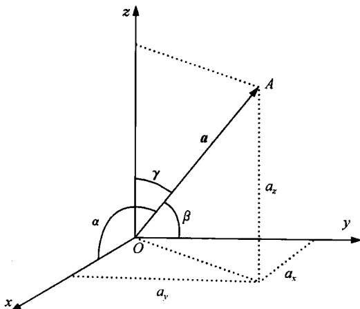
图 1.1 直角坐标系中的矢量 \mathbf{a}
