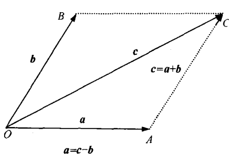
图 1.2 矢量相加(减)的平行四边形法则
