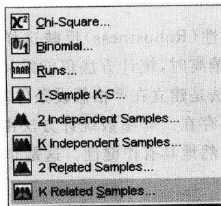
图 1.3 Nonparametric Tests 下拉菜单
