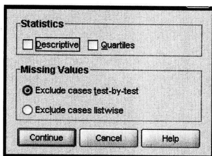
图 1.5 Options 对话框
