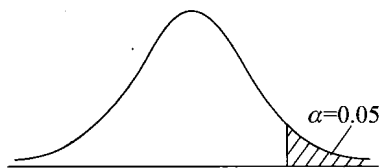
1.1 \alpha=0.05 的单侧检验否定域
