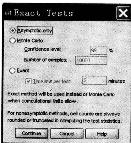
图 1.4 Exact Tests 对话框
