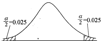
图 1.2 \alpha=0.05 的双侧检验否定域
