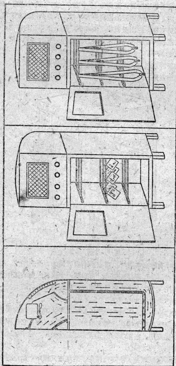
图 4. 干燥器构造图
