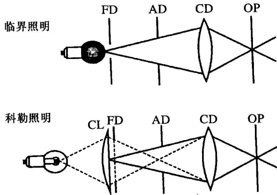
图 1-2 临界照明和科勒照明(引自林加涵等) CL 集光器; FD 视场光阑; AD 孔径光阑; CD 聚光器; OP 载物台
