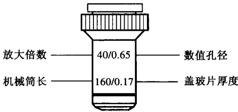
图 1-5 物镜的性能参数
