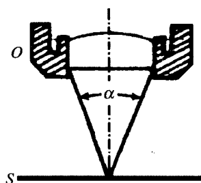
图 1-3 物镜的镜口角 O 物镜；S 标本； \alpha 镜口角
