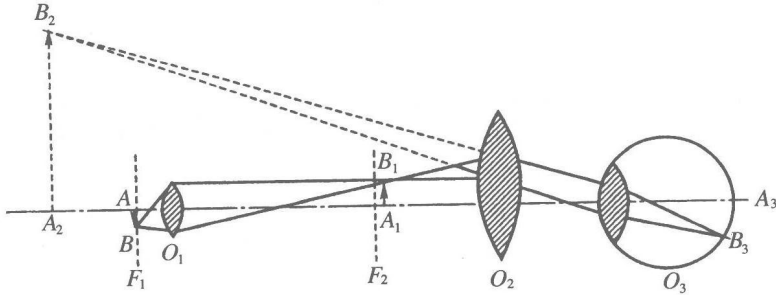
图 1-1 光学显微镜的放大原理和光路图(引自汪德耀) O_1 物镜; O_2 目镜; O_3 眼球; F_1 物镜的前焦点; F_2 目镜的前焦点
