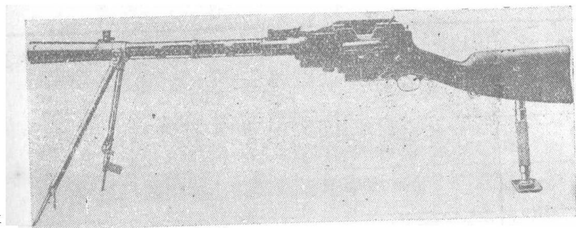
第 8 圖 德國最新式的輕機關槍
