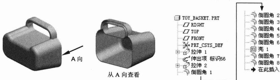
图 2.1 零件模型及模型树
