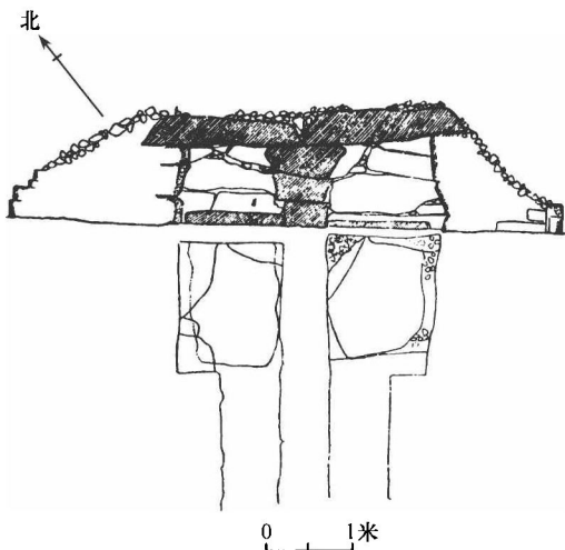
图三 第31号墓平、剖面图
