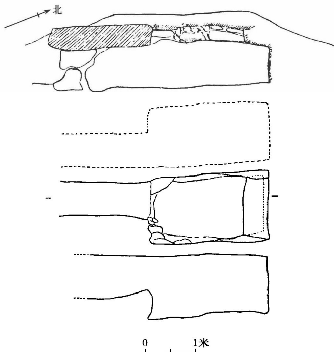
图四 第21号墓平、剖面图
