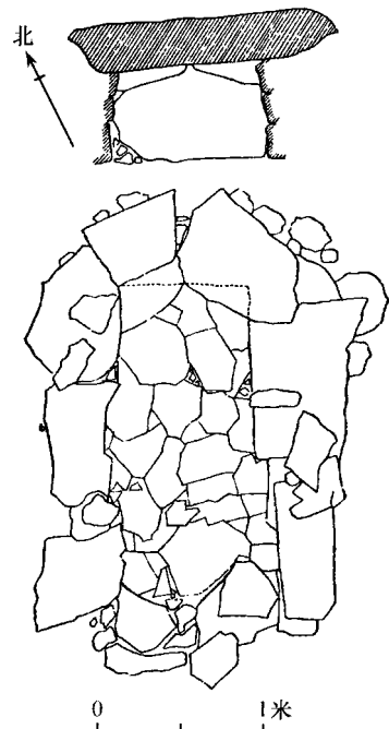
图五 第 43 号墓平、剖面图
