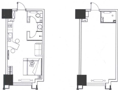
平面布置图
