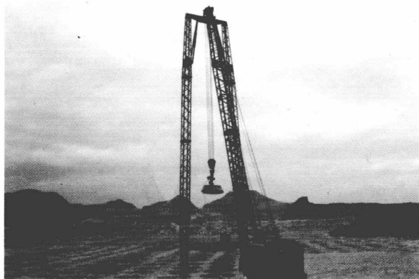
强夯机正在夯实跑道地基
