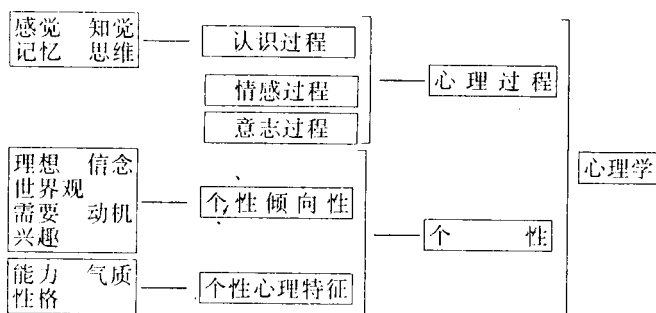
图 1-1 心理学内容结构
