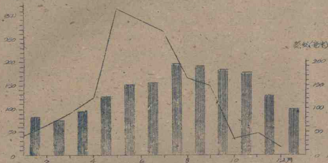
1951-1953年逐月平均降水量、蒸发量分布图
