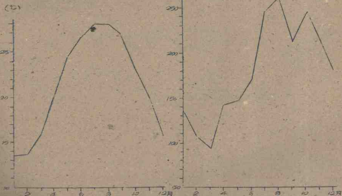
1951-1953年逐月平均气温分布图
