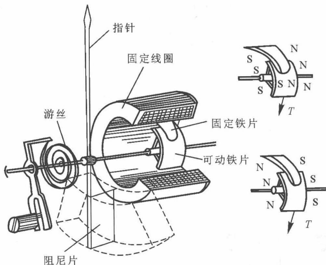
图 2-8 排斥型电磁系仪表测量机构
