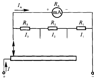
图 2-5 环形分流器
