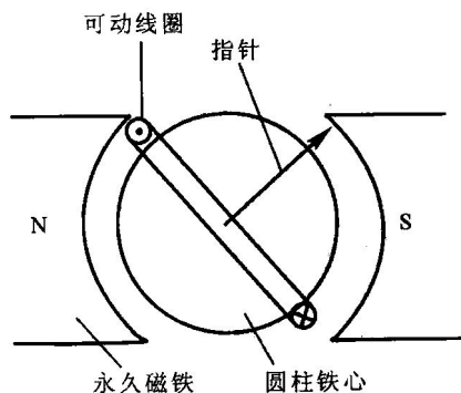
图 2-2 磁电系仪表工作原理
