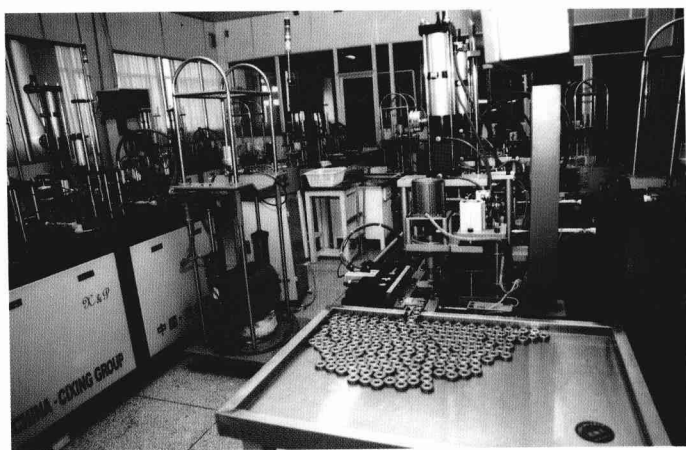
轴承自动总装线一角
