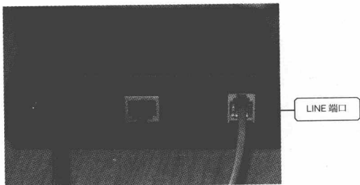
③ 在 ADSL Modem 上一般有两个连接端口, 分别是 LINE 端口和 LAN 端口。利用一根电话线将信号分离器的“Modem”端口与 ADSL Modem 的“LINE”端口连起来, 如图 1-7 所示。
