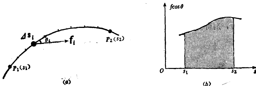
图 1-5 变力的功
