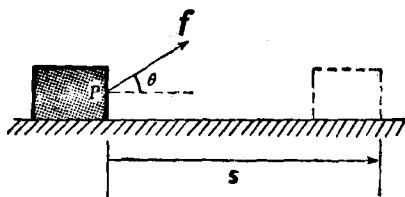
图 1-4 恒力的功
