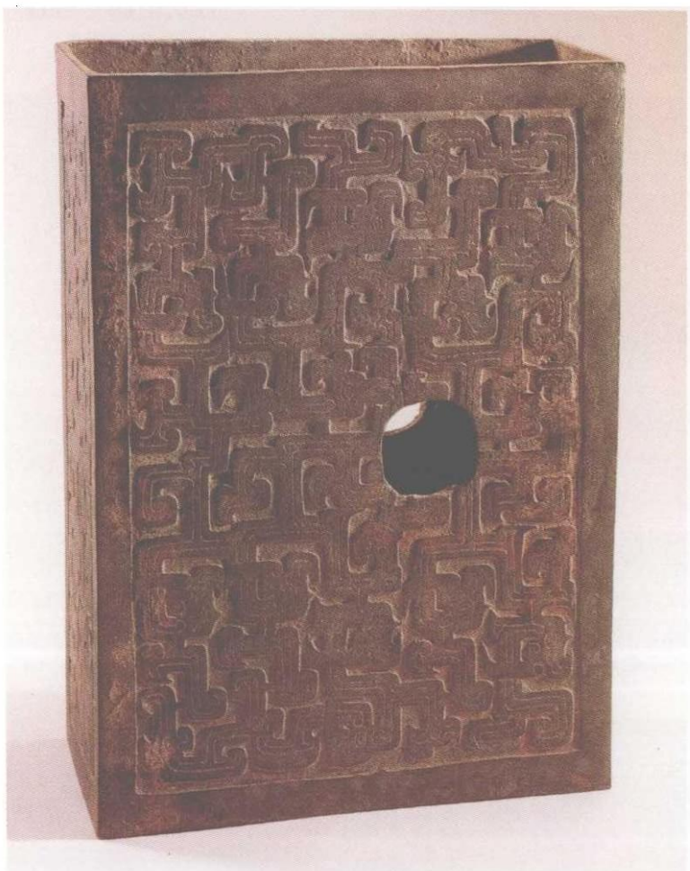
春秋中期 蟠蛇纹楔形 建筑构件
