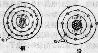
图1—2 原子结构示意图
