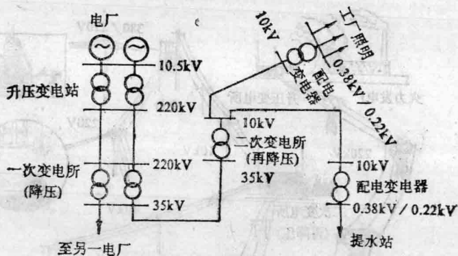
图1—4 电力系统原理性接线图
