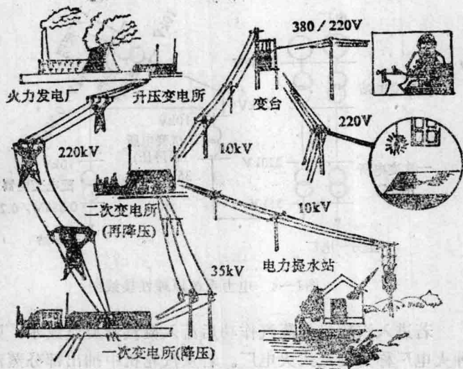
图1—3 电力系统示意图
