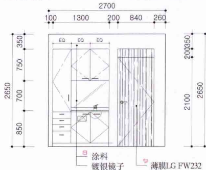
手术室立视图 C/elevation C(operation room)
