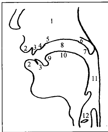
图 1 发音器官图
