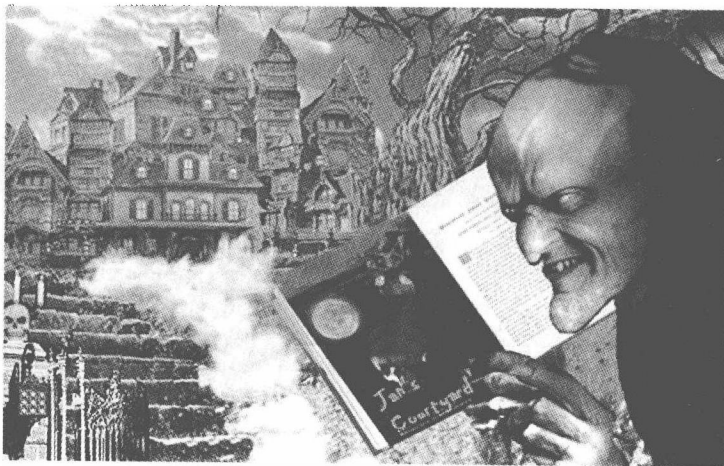
“凶宅”现象与重金属、放射性元素有关
