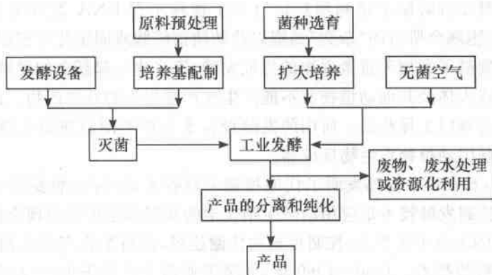
图 1-1 发酵工业工艺流程简图
