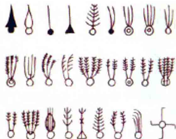
◇湖南长沙马王堆汉墓出土的帛书里对彗星的描绘。
