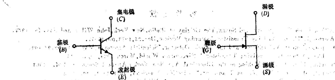
图1-6 NPN双极结型晶体管（BJT）的电符号
