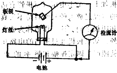
图1-1 爱迪生效应
