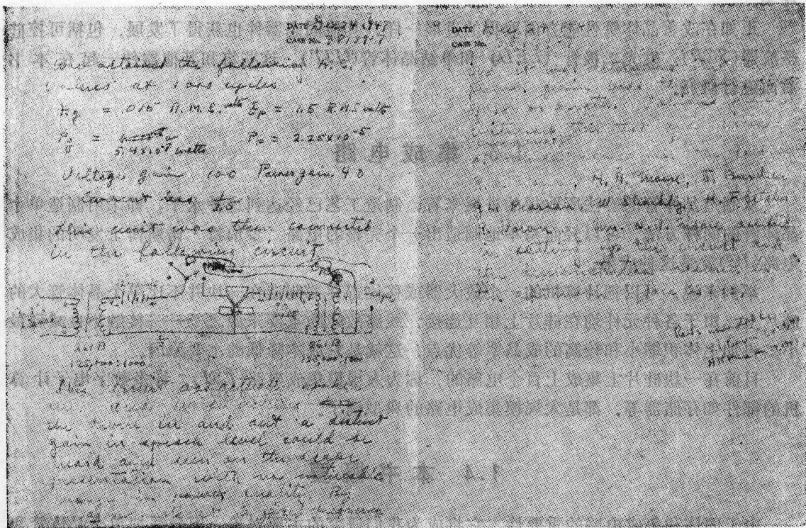
图1-5 这一页实验记录写下了1947年12月24日发现晶体管效应时的实验结果（承蒙贝尔电话实验室供稿）
