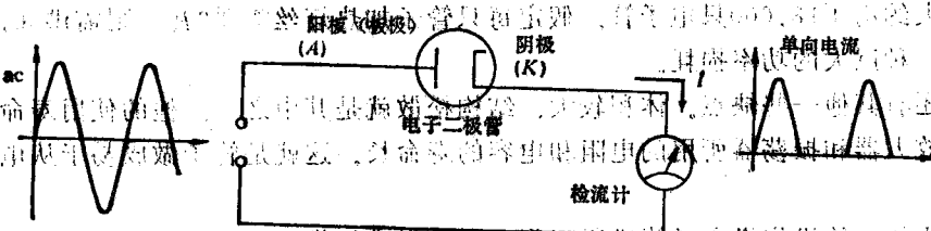
图1-2 用电子二极管把交流电流转换成单向电流
