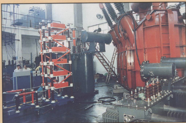
兴宁市电力集团公司变压器厂产品——大容量 有载调压节能变压器
