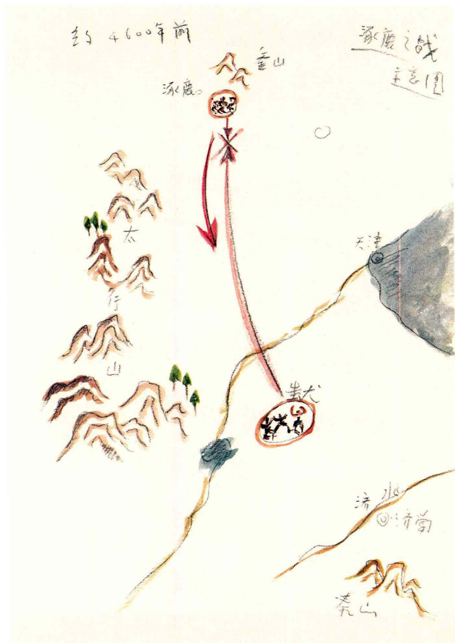
涿鹿之战
