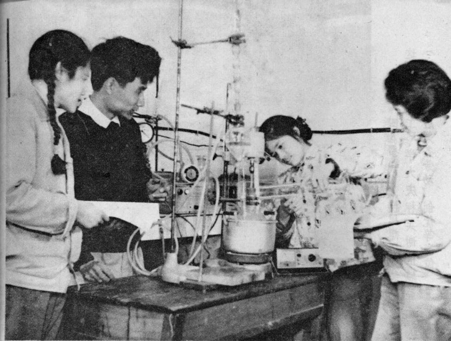
柳州地区六塘农药厂马拉松三结合攻关小组，为制造更优质价廉的农药，正在进行原料代用试验。
