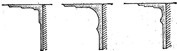
图 1 平顶阶梯形、曲面形线脚
