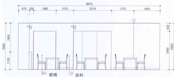
大厅立视图 /elevation(hall)
