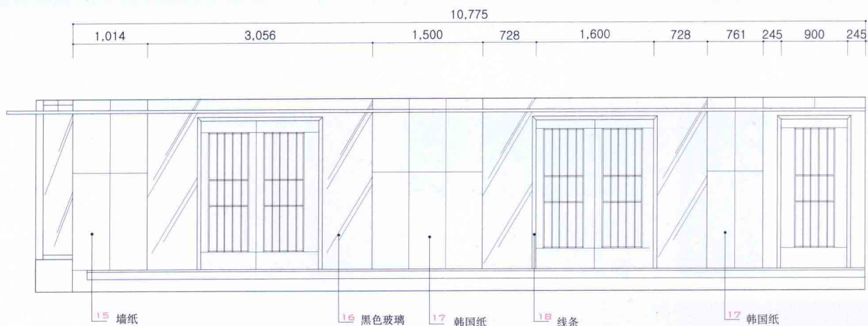
走廊立视图/elevation(corridor)
