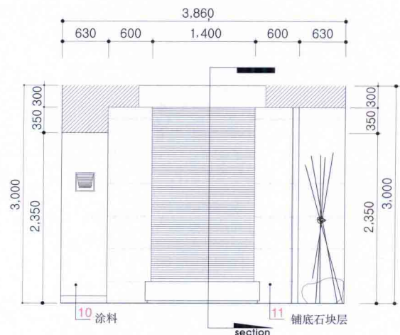
入口立视图 / elevation A (entrance)
