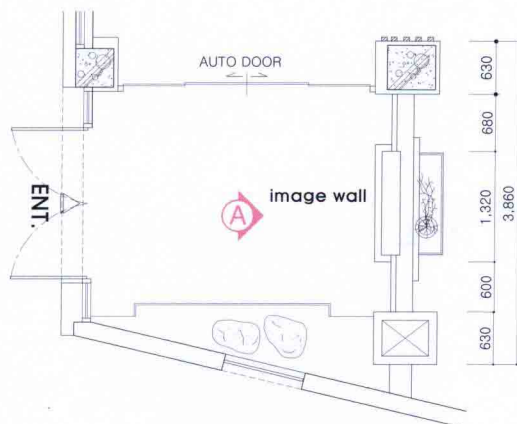
入口地面平面图 / floor plan (entrance)
