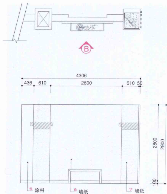
立视图 B/elevation B
