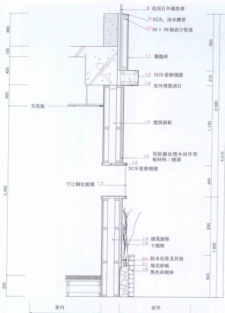
固定座椅详图 /detail(fixture chair)
