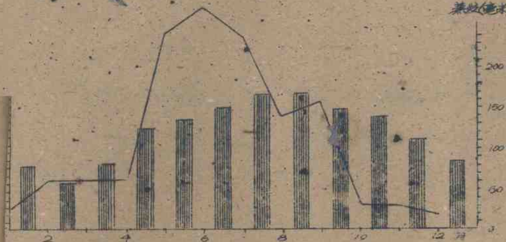
1955—1958年逐月平均降水量、蒸发量分布图
