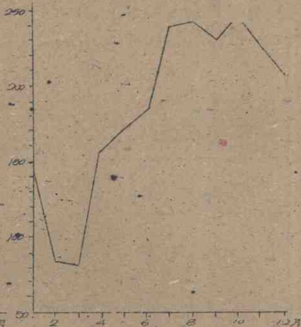
1955—1958年逐月平均日照时数分布图
