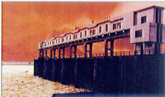
■ 改建后的赣抚平原焦石坝枢纽工程
