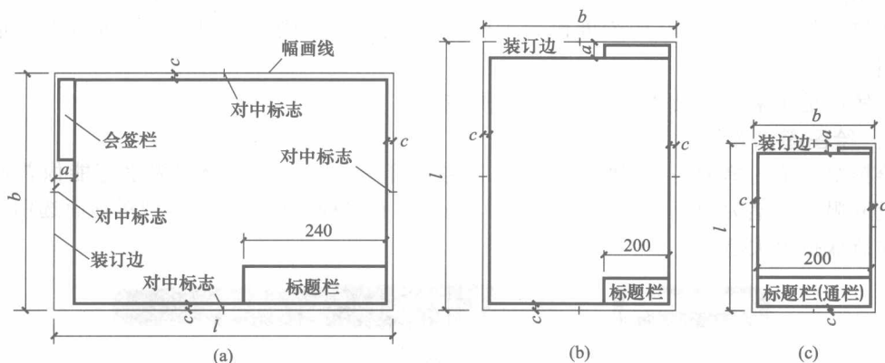
图 1-11 图幅格式
