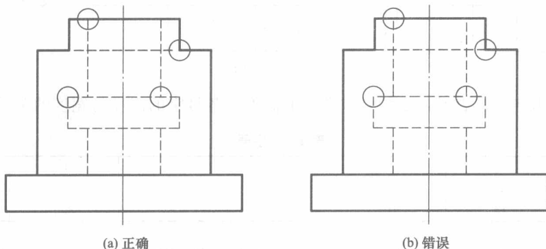
图 1-15 虚线交接的画法
