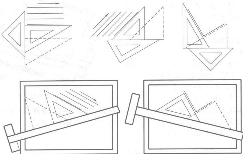
图1-4 用三角尺画平行线及垂直线
