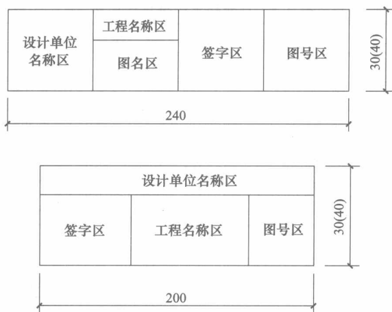
图 1-12 图标
