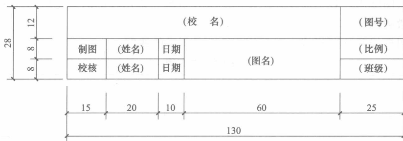
图 1-14 学生制图作业用标题栏推荐的格式
