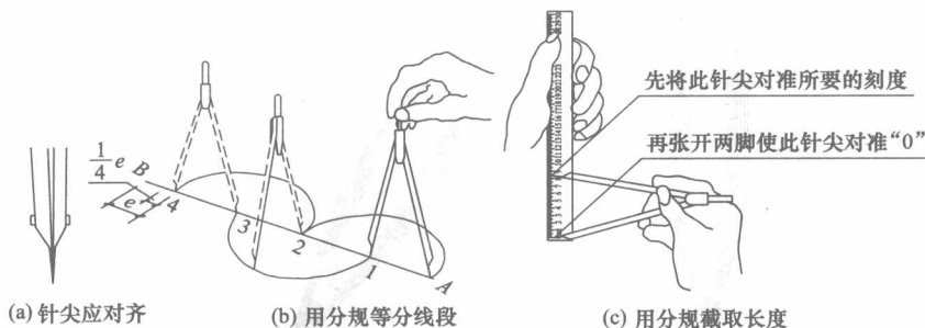
图 1-7 分规的用法
