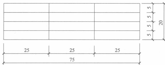
图 1-13 会签栏
