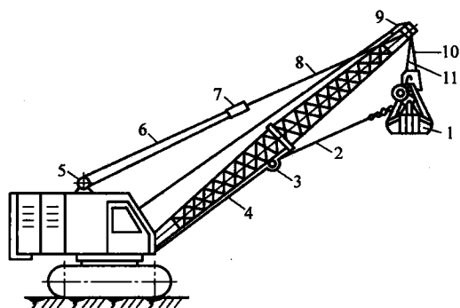
图 1-3 抓铲挖掘机
