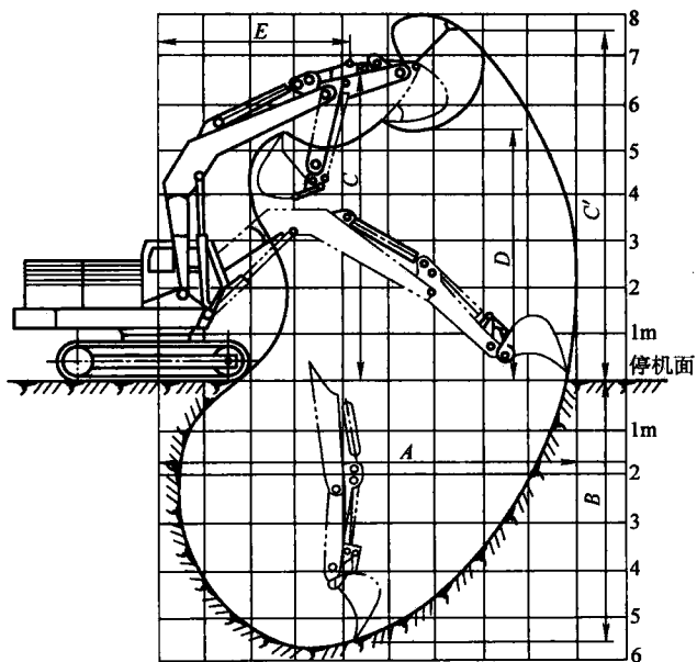
图 1-4 单斗反铲液压挖掘机的挖掘图
