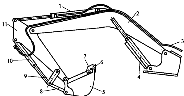
图 1-5 反铲
