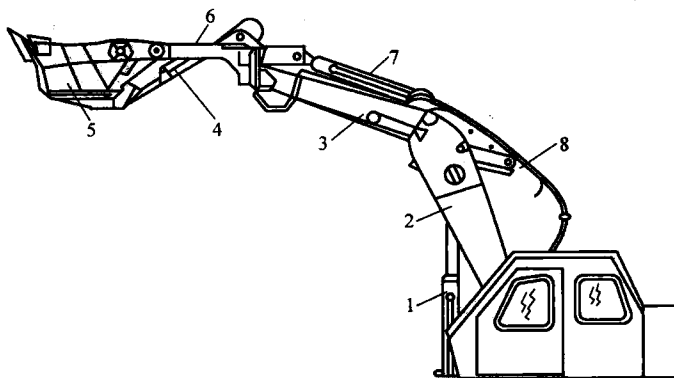
图 1-9 正铲 1—动臂液压缸 2—动臂 3—加长臂 4—斗底液压缸 5—铲斗 6—斗杆 7—斗杆液压缸 8—液压软管
