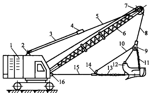
图 1-2 拉铲挖掘机
