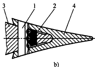
图 1-8 斗齿安装型式 a) 螺栓联接 b) 橡胶卡销联接 1—卡销 2—橡胶卡销 3—齿座 4—斗齿
