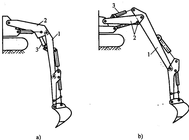
图 1-6 组合式动臂
