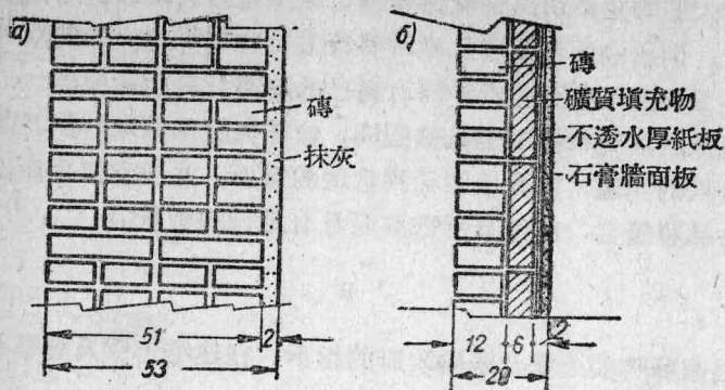
圖1 磚牆
