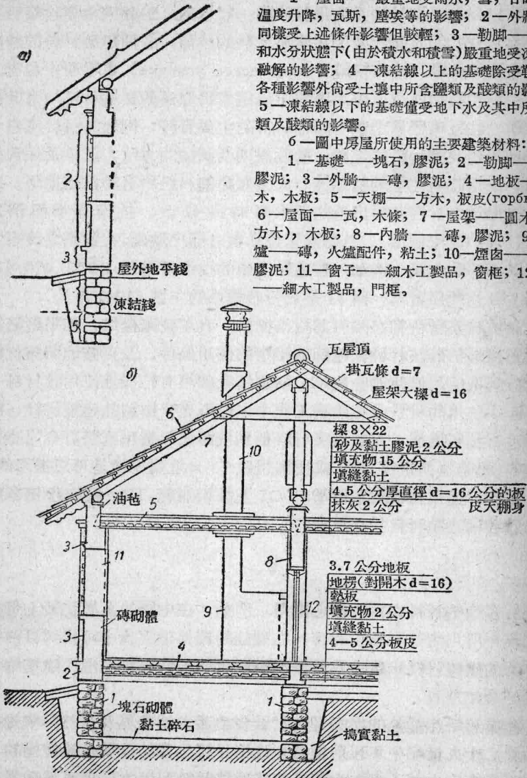
圖 2 住宅剖面圖的一部分
