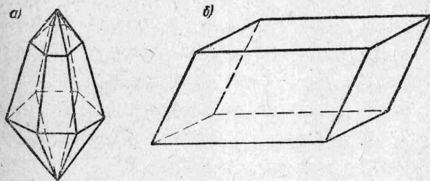
圖3 晶體的形狀
