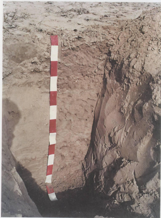
砂质潮土剖面 (郑州市东郊廿里铺)
