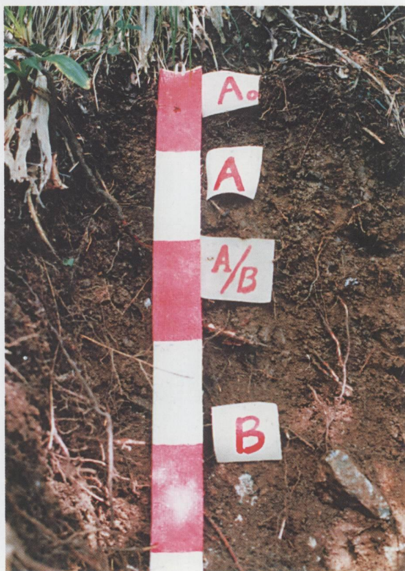
棕壤剖面 (栾川县老君山)
