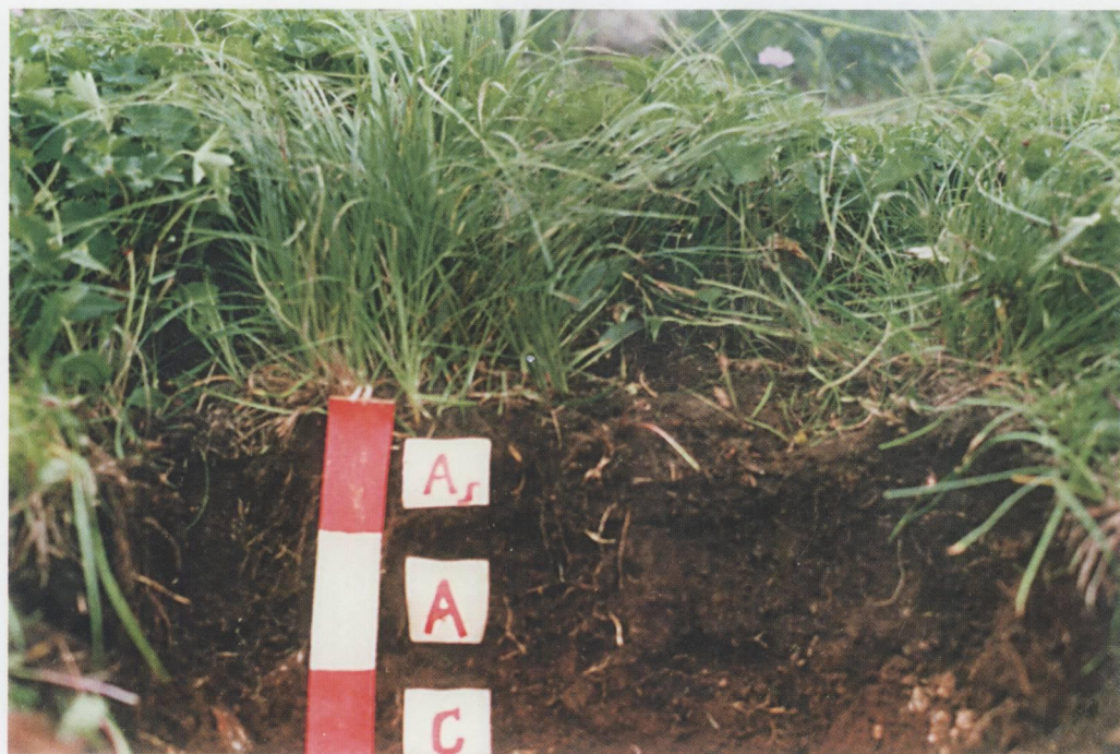
山地草甸土剖面 (栾川县老君山顶亮宝台 2160m)
