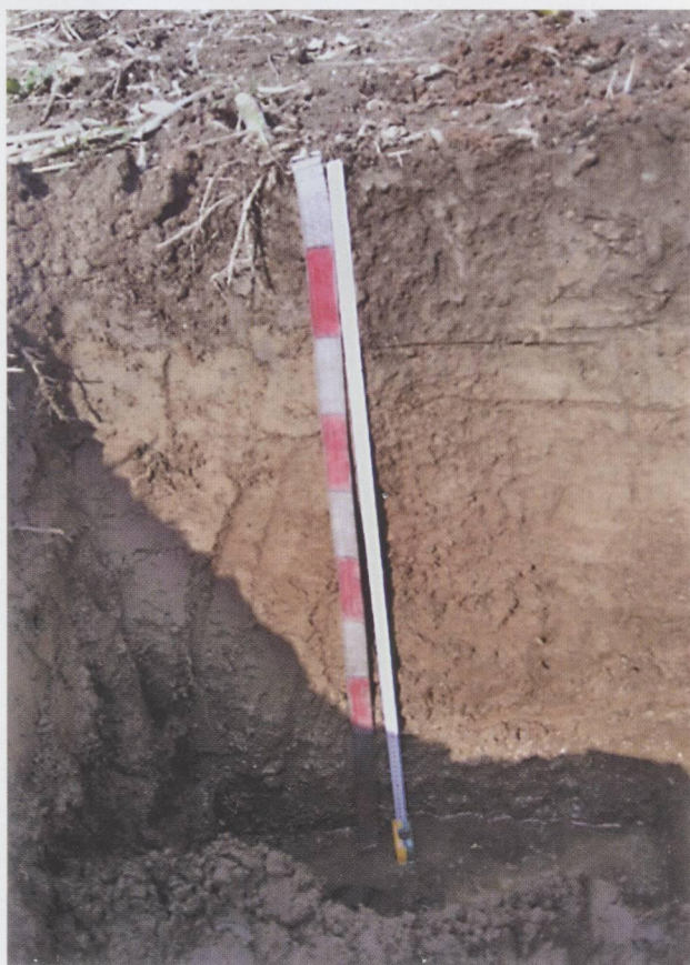
壤质潮土剖面 （开封市郊区）
