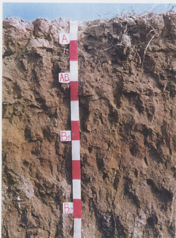
褐土剖面（陕县张村塬）
