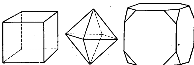
(a) 立方体
