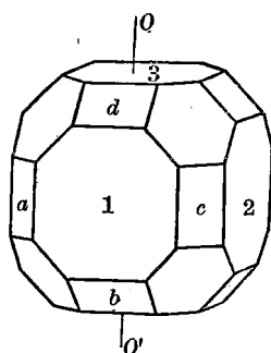
图 1-1 晶体外形图
