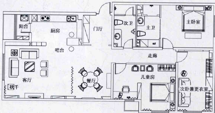
平面布置图
