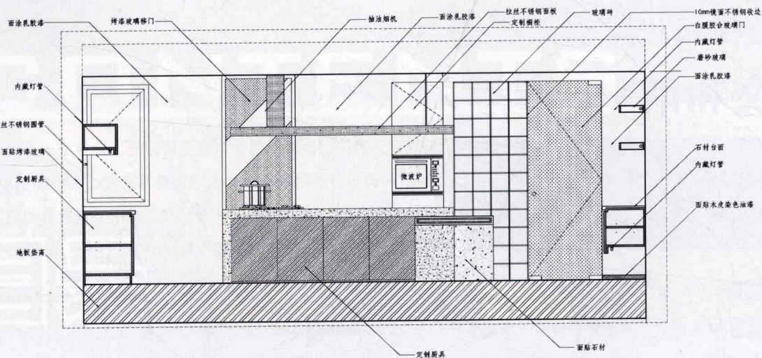
厨房立面设计图
