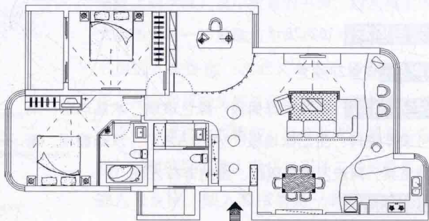
平面布置图
