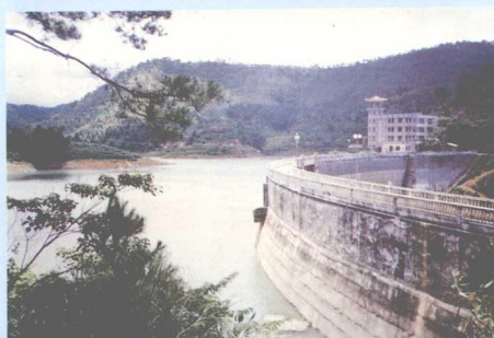
北流大村双曲拱坝
