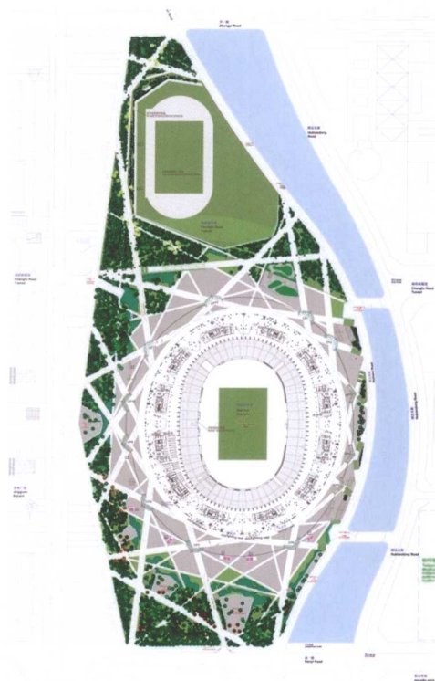
设计总平面图
