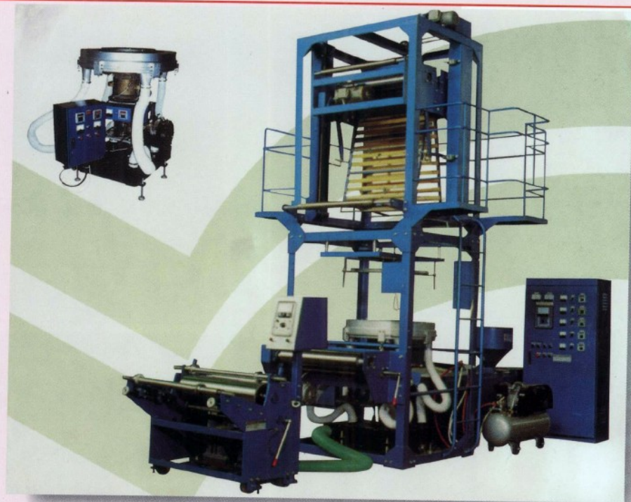
▲ 汕头机械集团公司的高低密度聚乙烯吹塑机组
