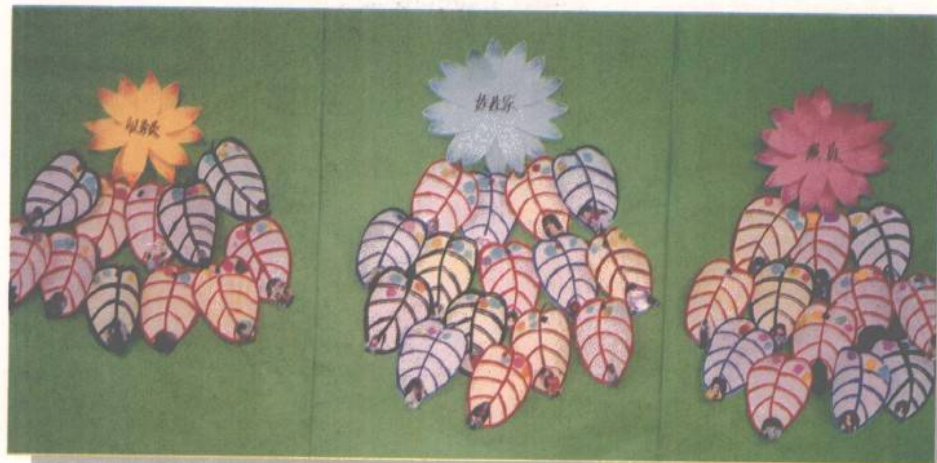
▲ 进区统计图
